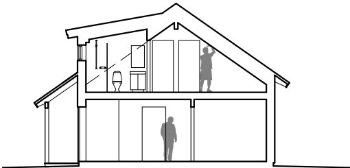
PRINCIPSNITT
