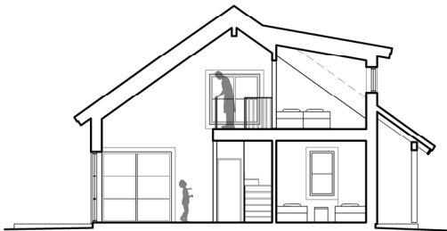
PRINCIPSNITT
